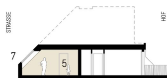
Schnitt 2 (schematisch)
