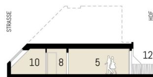
Schnitt (schematisch)
