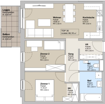
2. Obergeschoß M: 1: 100
