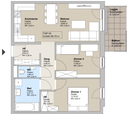
2. Obergeschoß M: 1: 100
