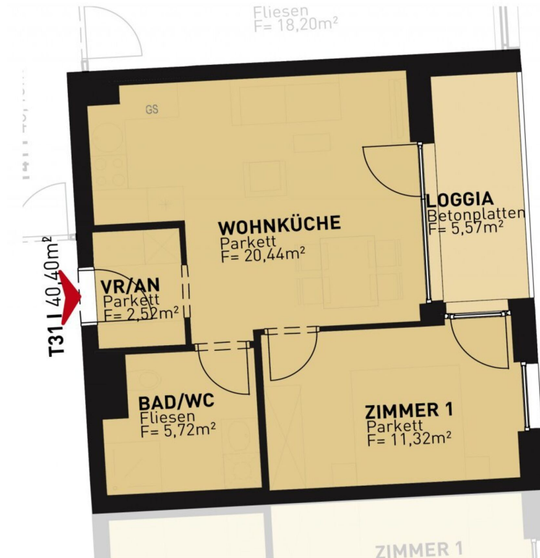
DRYGALSKIWEG 59 | 1210 WIEN — 2. OBERGESCHOSS ↑ NORDEN
