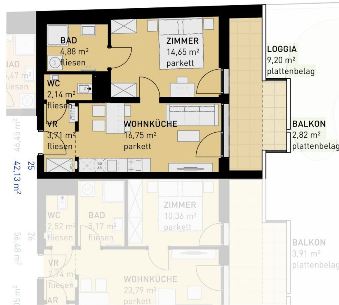
STUDENYGASSE 16 | 1110 WIEN 1. OBERGESCHOSS
