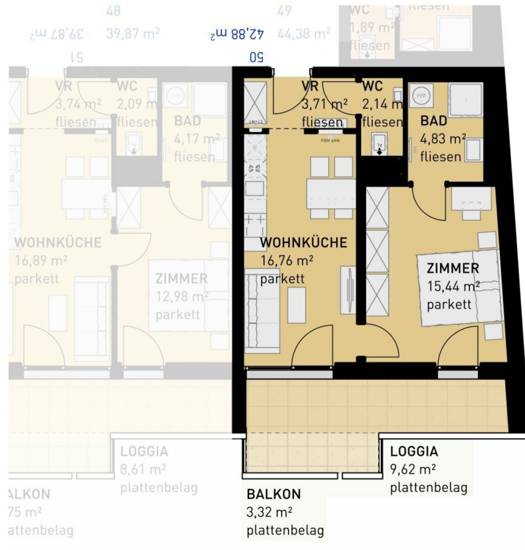
STUDENYGASSE 16 | 1110 WIEN 2. OBERGESCHOSS
