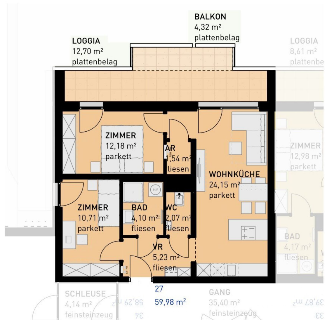
STUDENYASSE 16 | 1110 WIEN 1. OBERGESCHOSS
