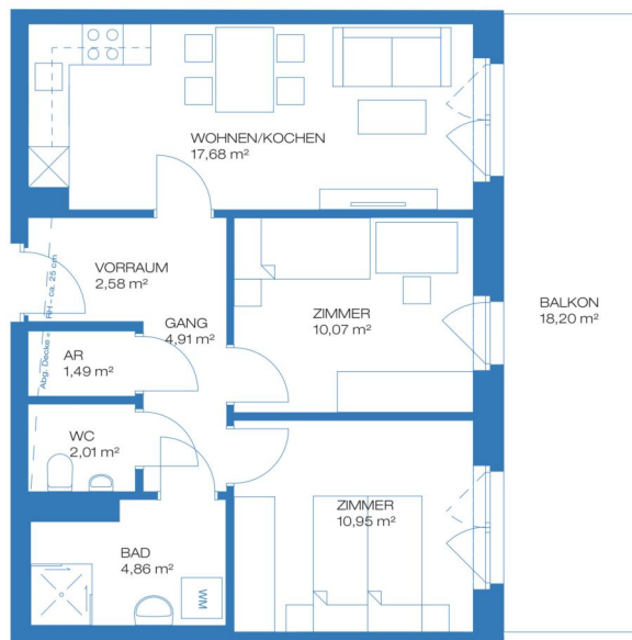
TOP 32, TYP C3 GESAMTFLÄCHE 54,55 m² AUßENBEREICHE Balkon 18,20 m²
