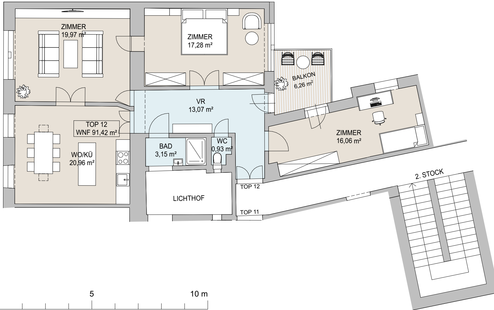
GRUNDRISS 1/100
