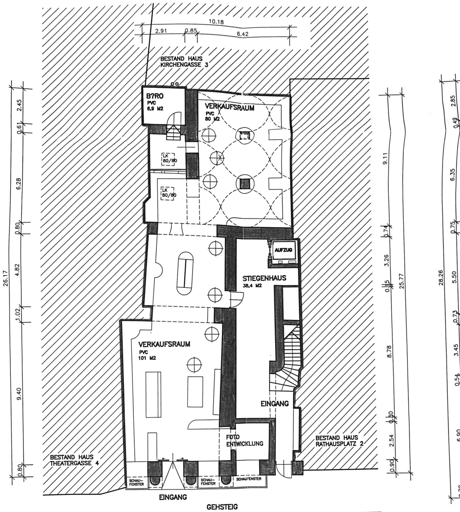
GRUNDRISS ERDGESCHOSS
