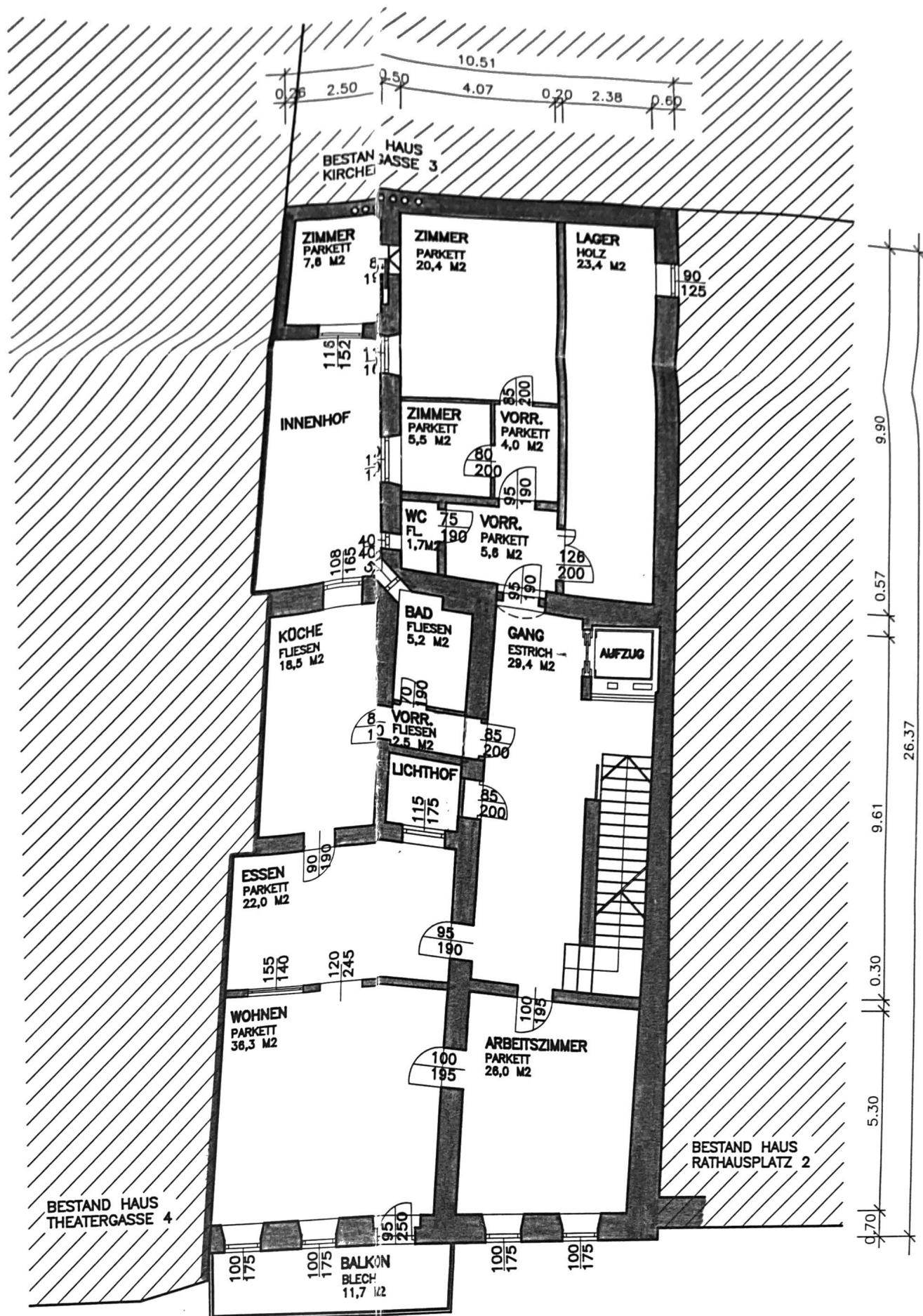
GRUNDRISS 2. OBERGESCHOSS
