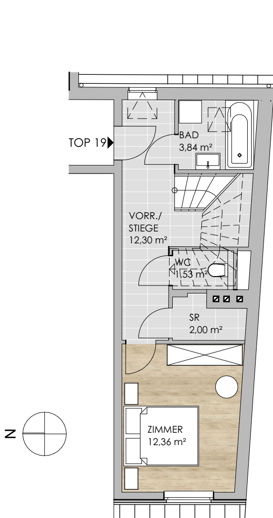
1.DACHGESCHOSS
