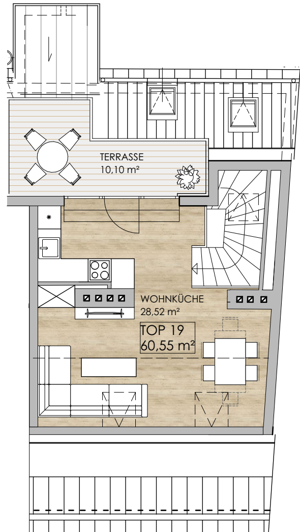
2.DACHGESCHOSS
