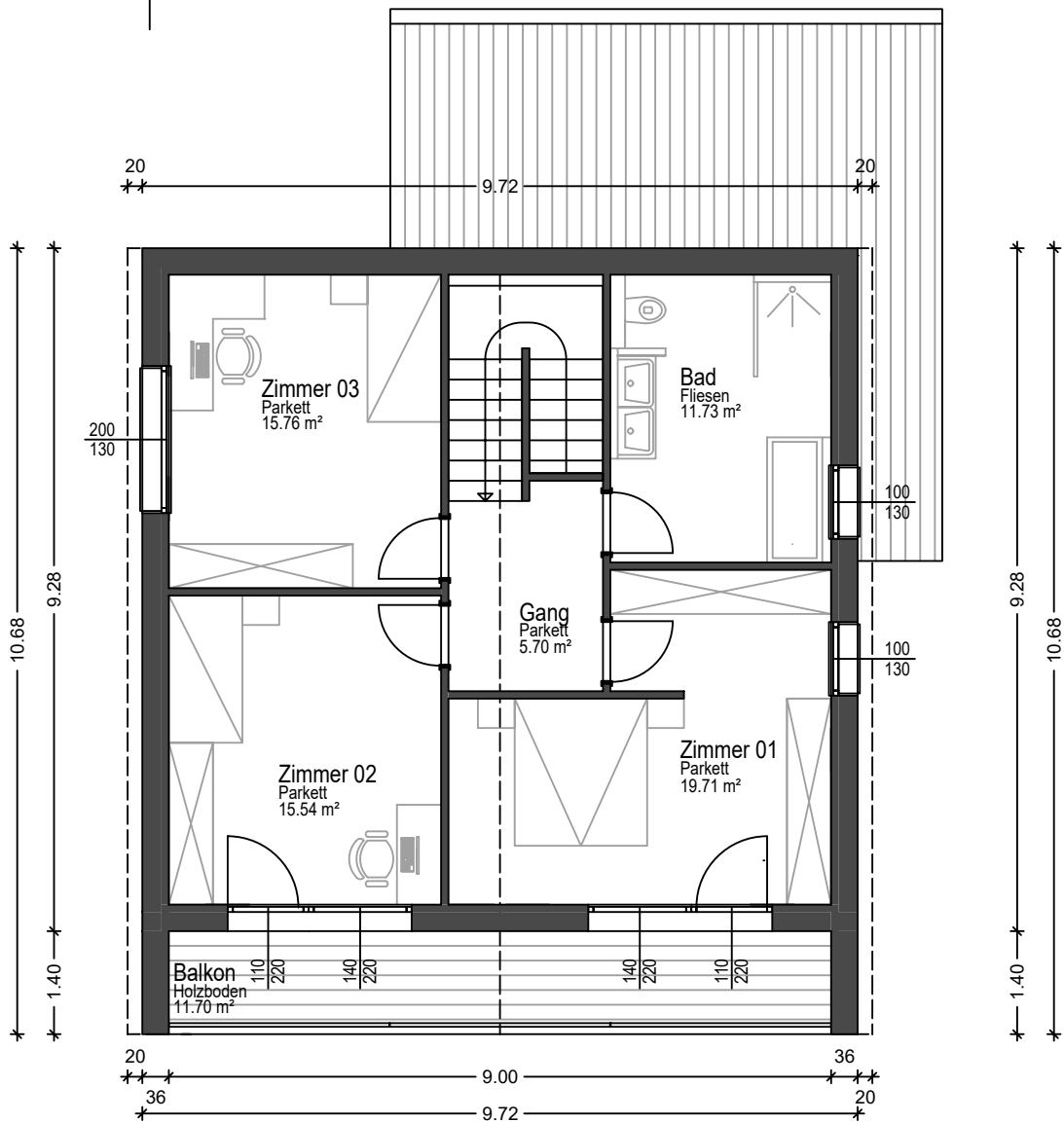
OBERGESCHOSS
