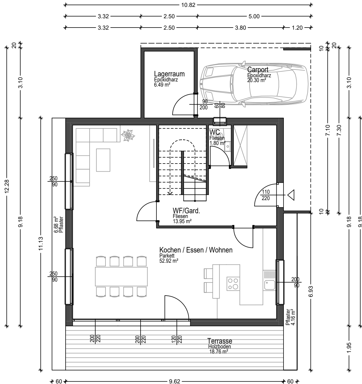
ERDGESCHOSS
