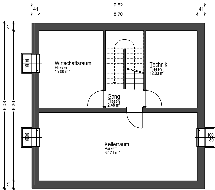
KELLERGESCHOSS
