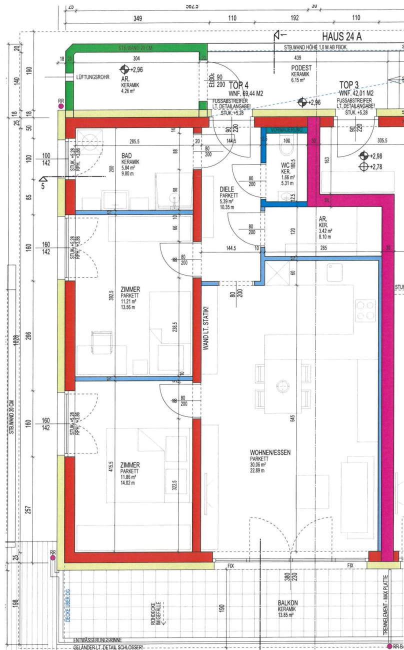
Haus A Wohnung TOP 4 - 1. OG
