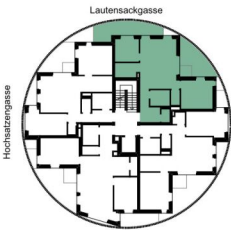
GESCHOßPLAN
