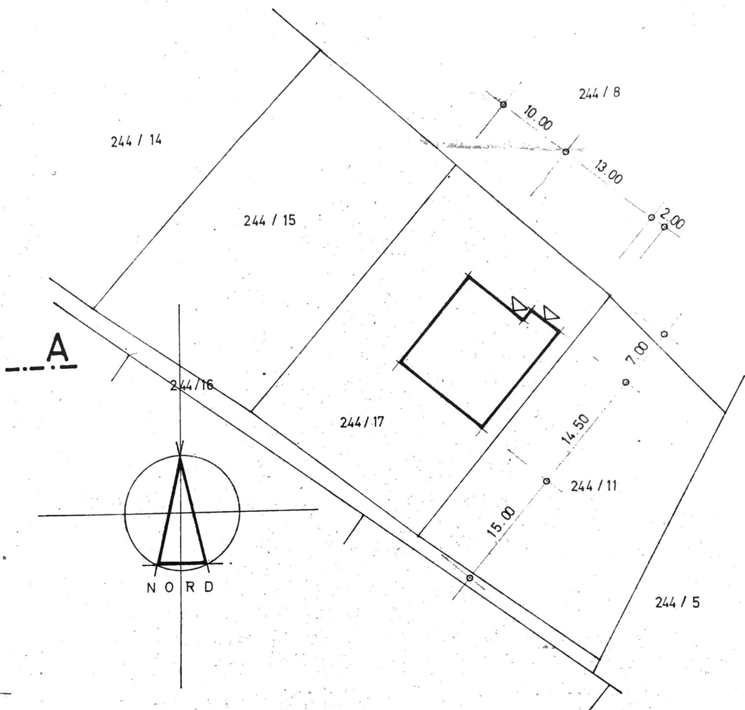
LAGEPLAN 1 : 500
