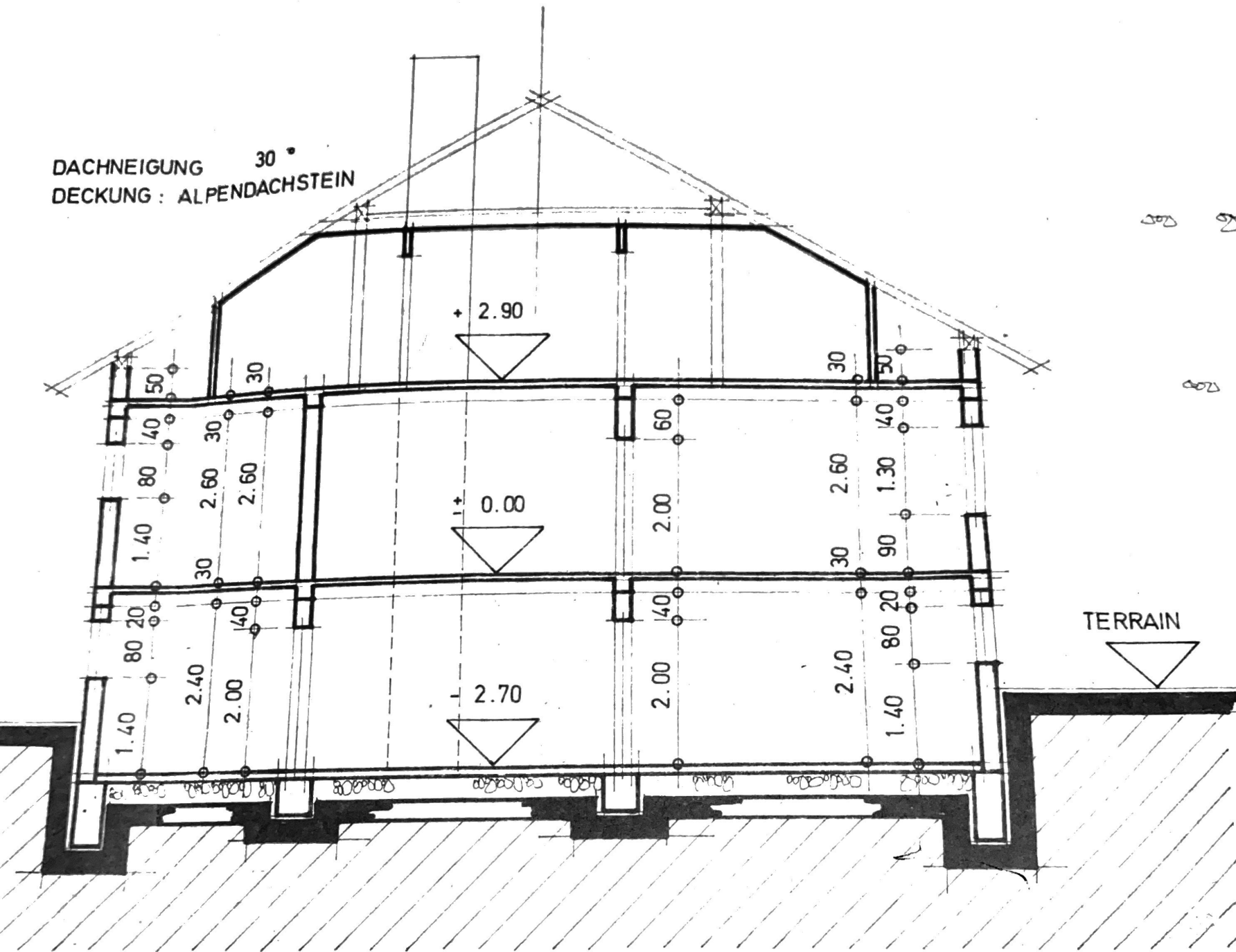
SCHNITT A-A
