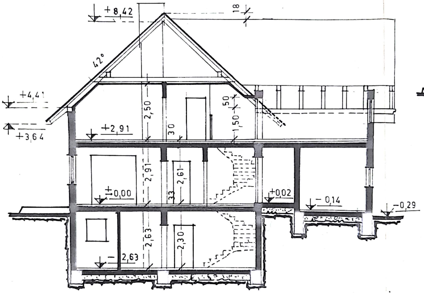
SCHNITT A-A
