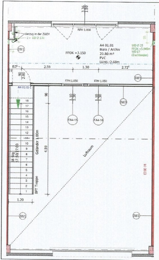
Obergeschoss
