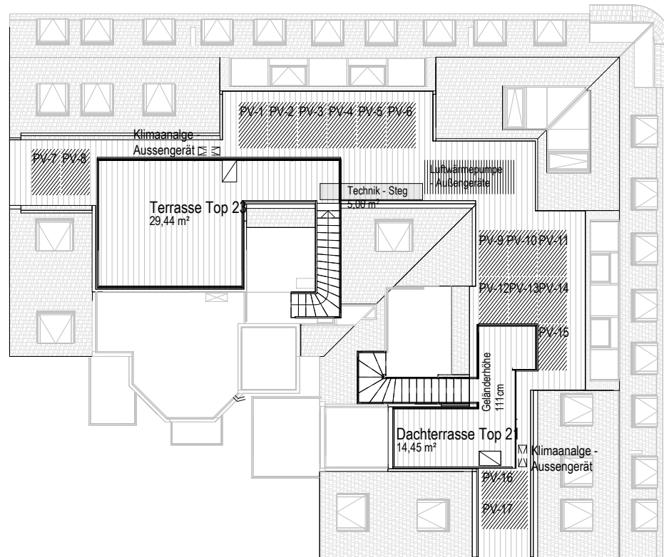
GR Dachdraufsicht
