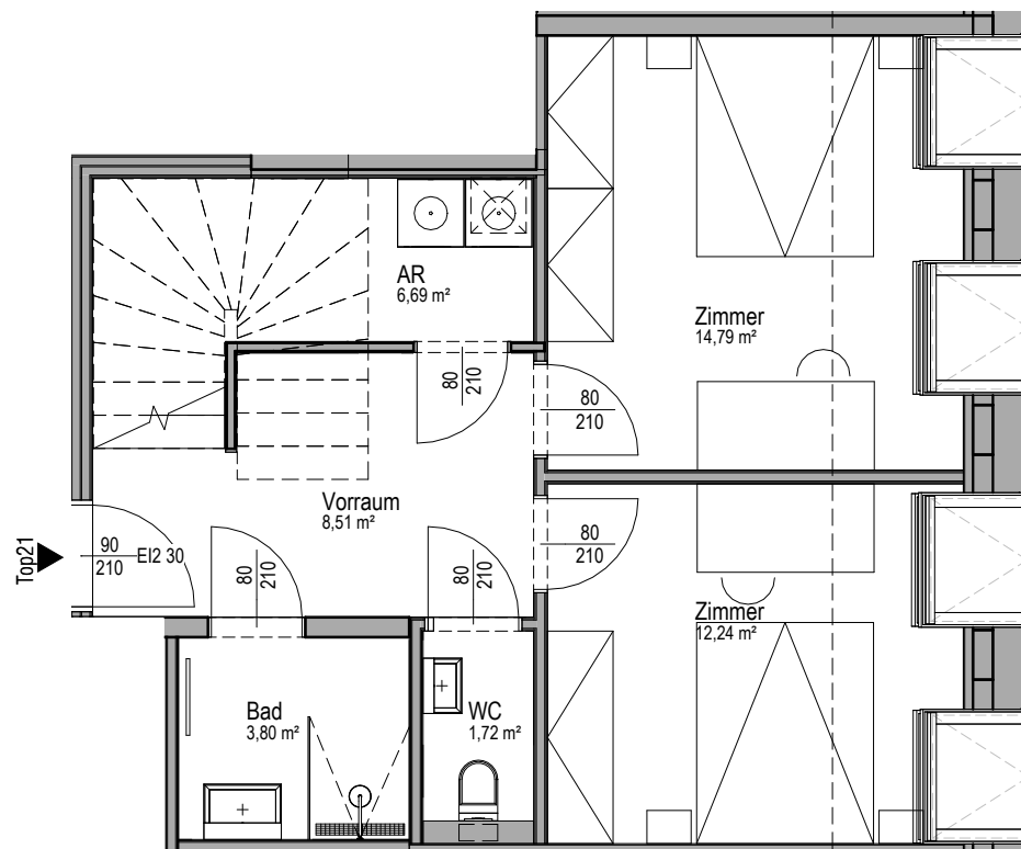
GR 1. Dachgeschoss
