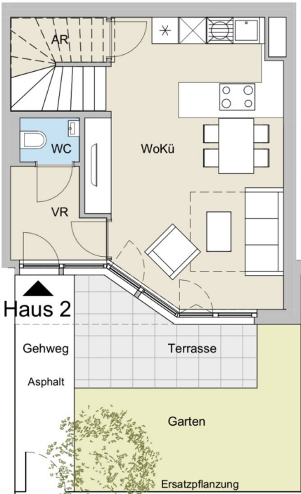
EG
