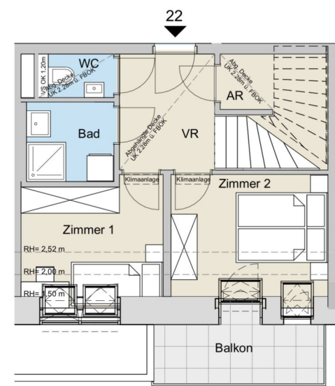
3. OG
