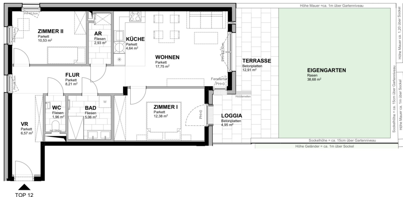
Übersichtsplan 1. Obergeschoss
