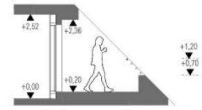
Schnitt 2
