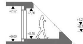
Schnitt 2
