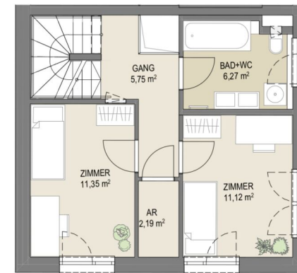
1. OG
