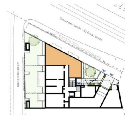
ORIENTIERUNGSPLAN | +0 ERDGESCHOSS
